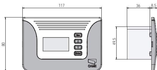
Mesures d'encombrement
